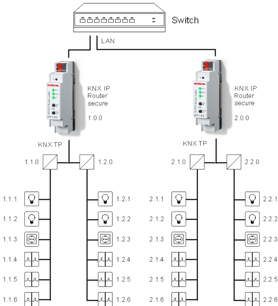
KNX IP Router als Bereichskoppler
