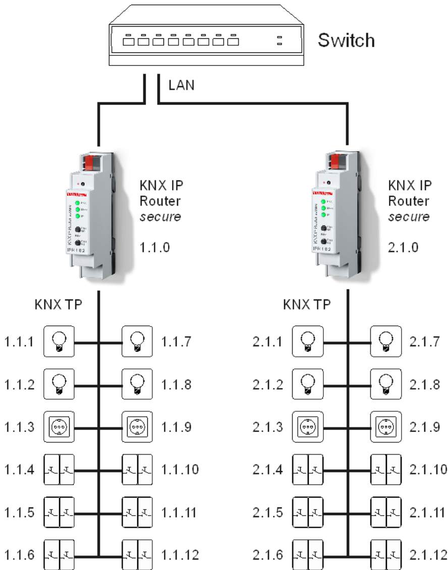
KNX IP Router als Linienkoppler
