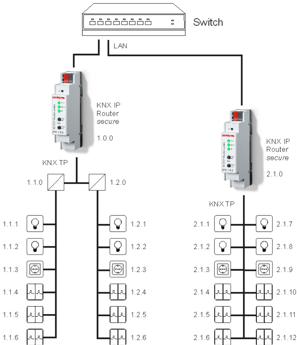
KNX IP Router als Bereichs- und Linienkoppler
